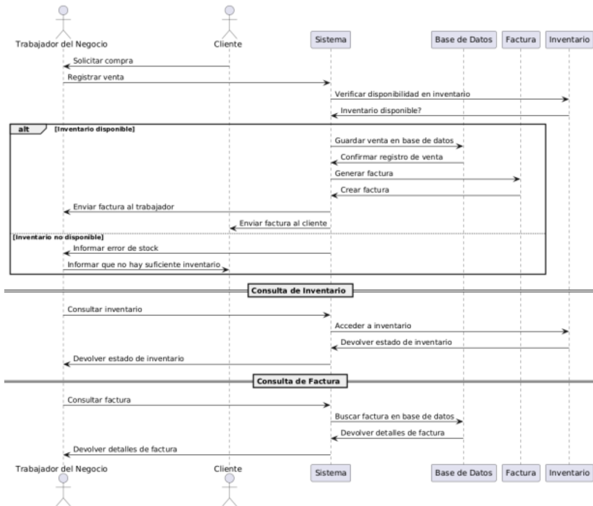
Diagrama de Secuencia, creado por el Alumno Deykert Guido, en donde se refleja el flujo de las acciones que podrá realizar el trabajador del Negocio.
